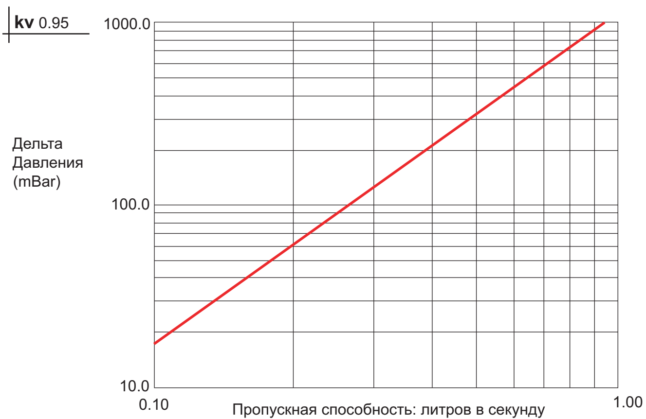
Диаграмма 981559/1: зависимость падения загрузки от пропускной способности магнитного противозвестного аппарата MiniElcla Ø 1/2" и 3/4".
